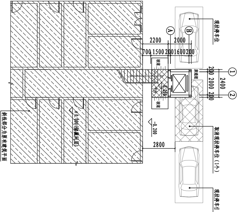
增设电梯后储藏间层平面图 1:150
